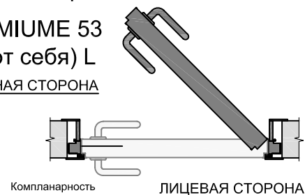
Вариант открывания "С"
