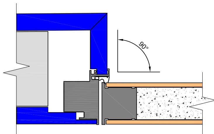
PREMIUME 40 OUT (на себя)
