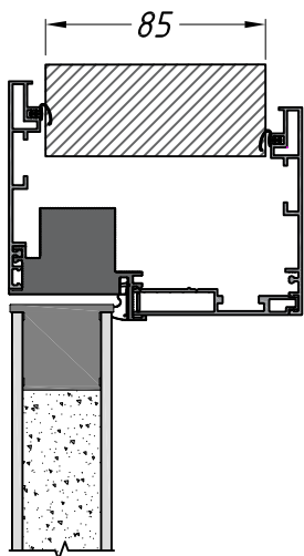
Один доборный ряд
