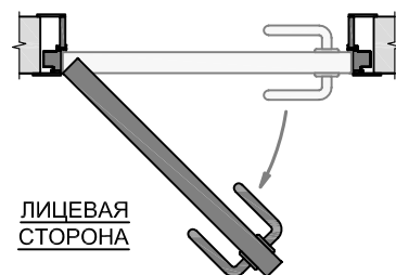
Вариант открывания "В" PREMIUME 40 OUT (на себя) L ОБРАТНАЯ СТОРОНА
