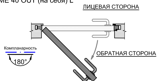
Вариант открывания "В" PREMIUME 40 OUT (на себя) L
